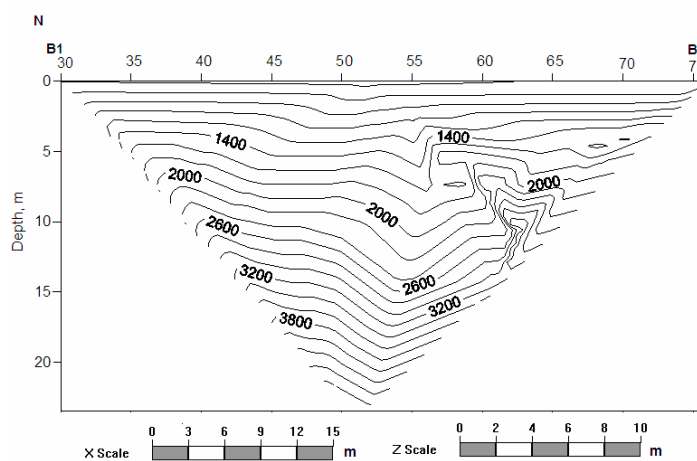
شکل ۵-۵- منحنی‌های میزان تغییرات سرعت با عمق
