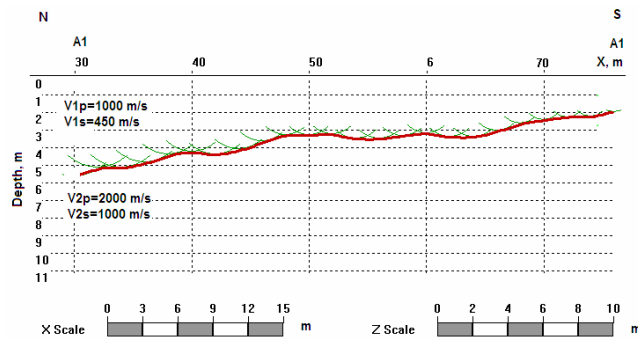
شکل ۴-۵- مقاطع لرزه‌ای شکست مرزی در محیط لایه‌ای
