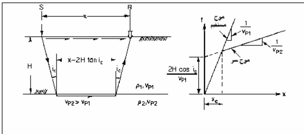
شکل ۲-۴ - مسیر پرتوها و منحنی‌های فاصله-زمان موج مستقیم و موج سر
