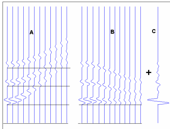
شکل ۴-۸-۱- نگاشت CDP در یک نقطه، B- نگاشت CDP بعد از تصحیح NMO، C- رد CDP
