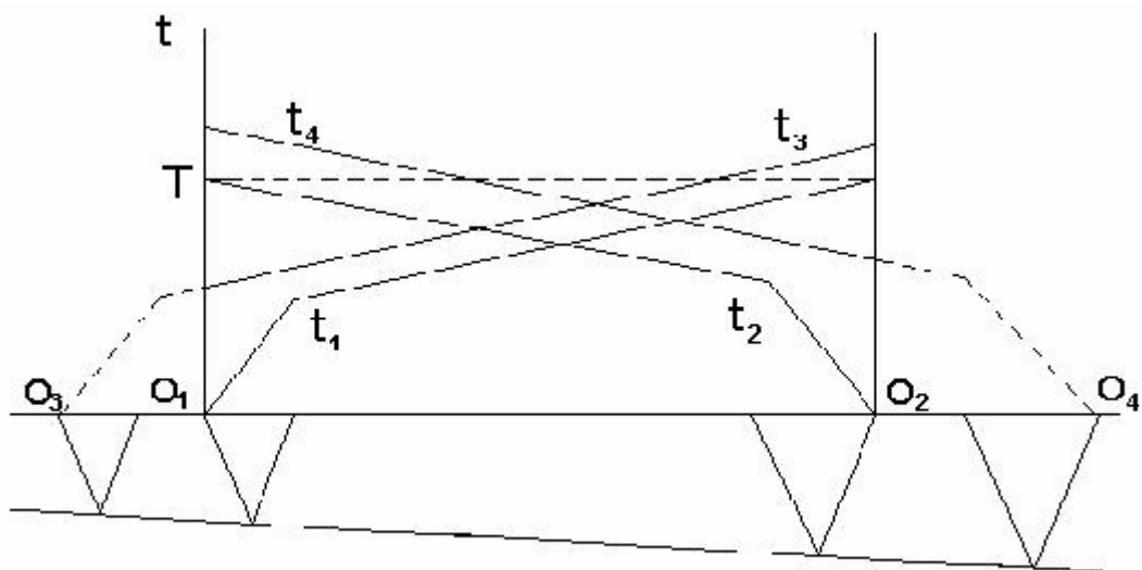
شکل ۴-۵- سیستم ۴ نقطه‌ای اجرای عملیات لرزه‌نگاری انکساری
